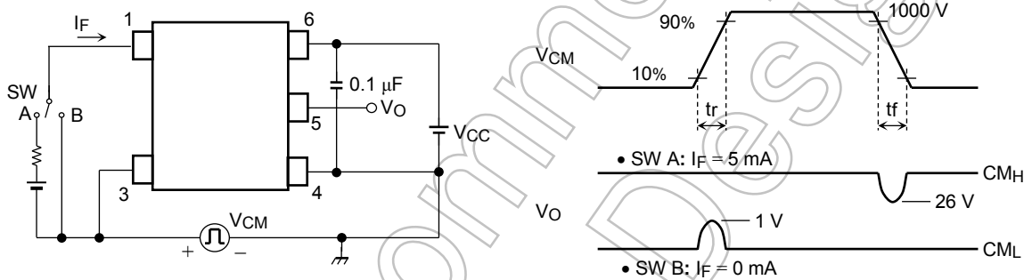
図 8 コモンモード過渡耐性測定回路、波形
