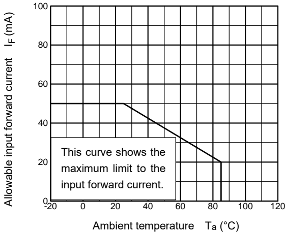
Fig.12.1 I_F - T_a
