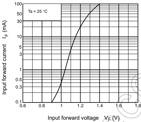
Fig.12.3 I_F - V_F
