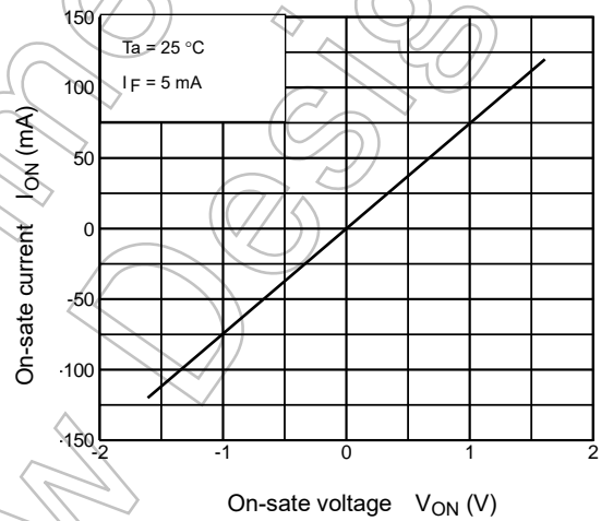
Fig.12.4 I_{ON} - V_{ON}
