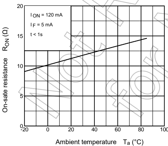
Fig.12.5 R_{ON} - T_a
