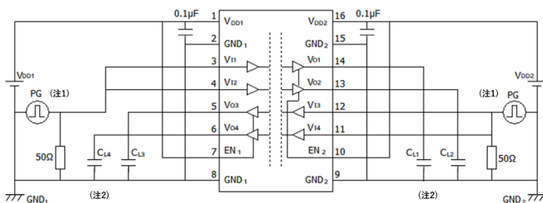
図 12-1-3: DCL342L0B/DCL342H0B Switching 特性測定回路図
