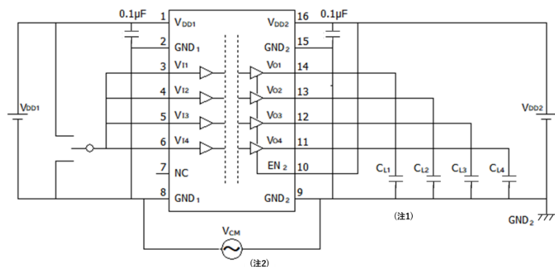
図 12-3-1: DCL340L0B/DCL340H0B コモンモード過渡耐性テスト回路図
