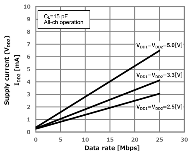
図 13.2. DCL340x0B I_{DD2} 動作電流—データレート
