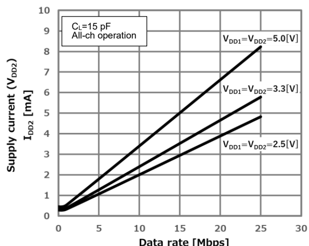
図 13.6. DCL342x0B I_{DD2} 動作電流—データレート
