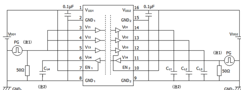
図 12-1-2: DCL341L0B/DCL341H0B Switching 特性測定回路図
