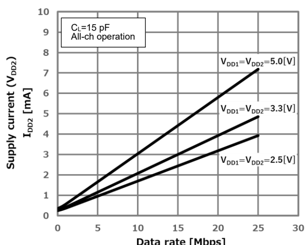
図 13.4. DCL341x0B I_{DD2} 動作電流—データレート
