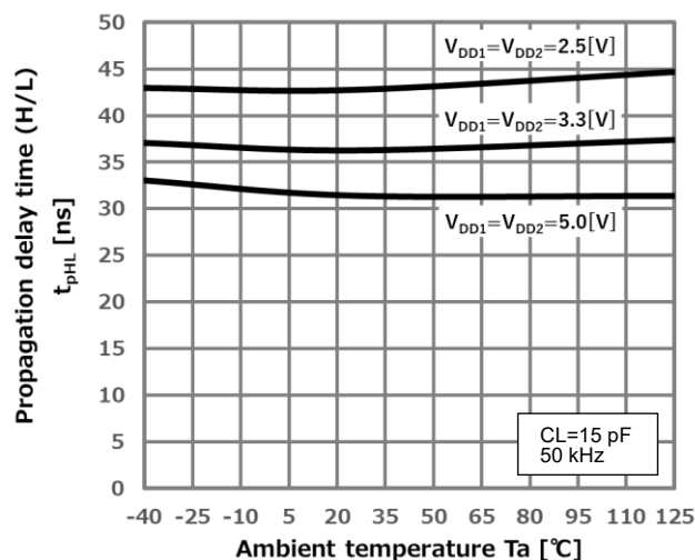
図 13.8. 伝搬遅延 t_{PLH} — T_a
