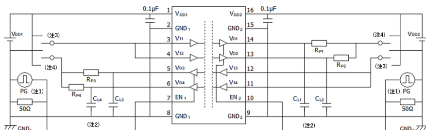
図 12-2-3: DCL342L0B/DCL342H0B イネーブル伝搬遅延時間テスト回路図
