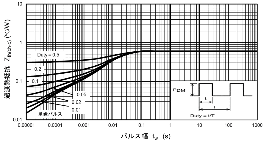
図 8.13 Z_{th(ch-c)} - t_w (最大値 (保証値))
