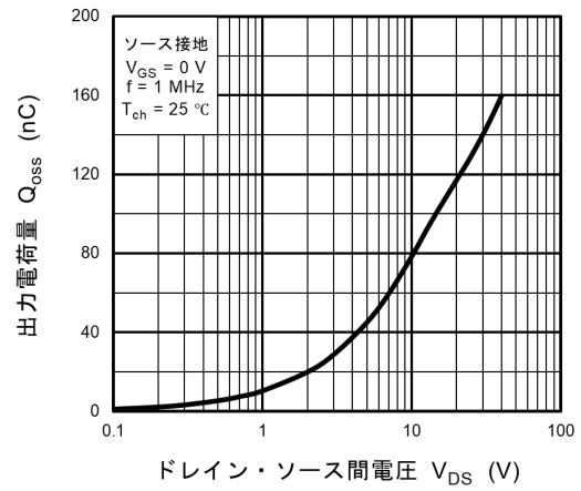
図 8.12 Q_{oss} - V_{DS}
