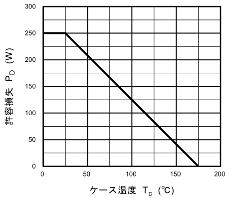
図 8.14 P_D - T_c (最大値 (保証値))
