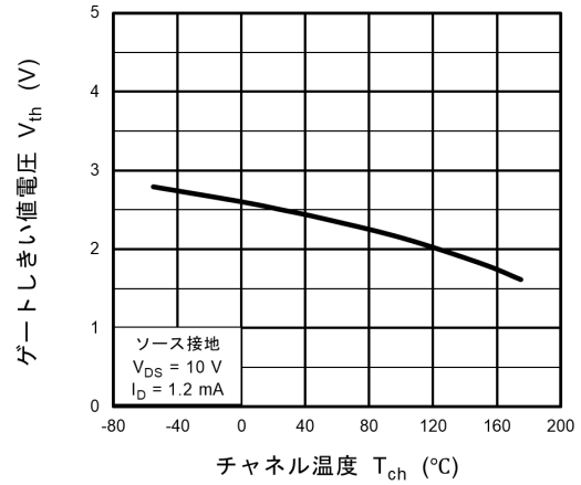
図 8.8 V_{th} - T_{ch}
