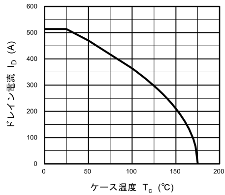
図 8.15 I_D - T_c
