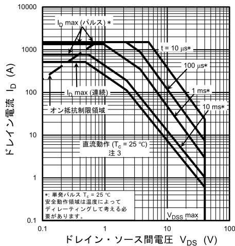
図 8.16 安全動作領域 (最大値 (保証値))
