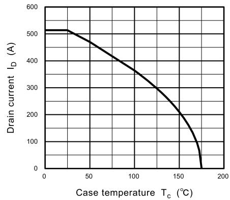
Fig. 8.15 I_D - T_c
