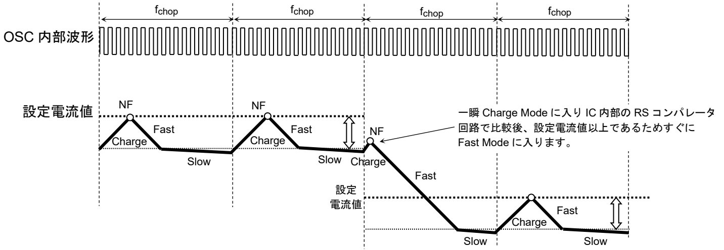
図 7.11 設定電流値が減少方向の場合
