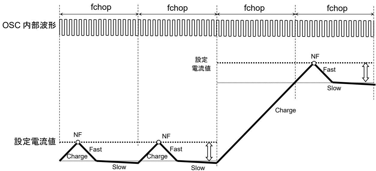
図 7.10 Charge 期間が fchop 1 周期以上の場合
