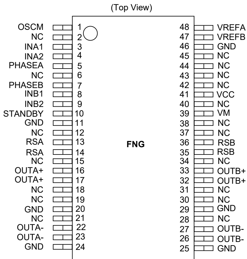
図 4.2 端子配置図 (TB67S101AFNG)
