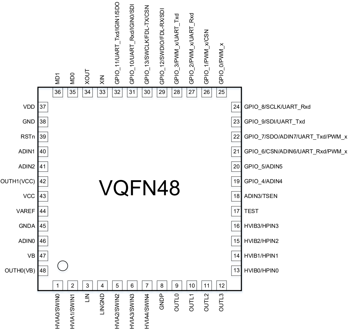
図 6.1 端子配置図
