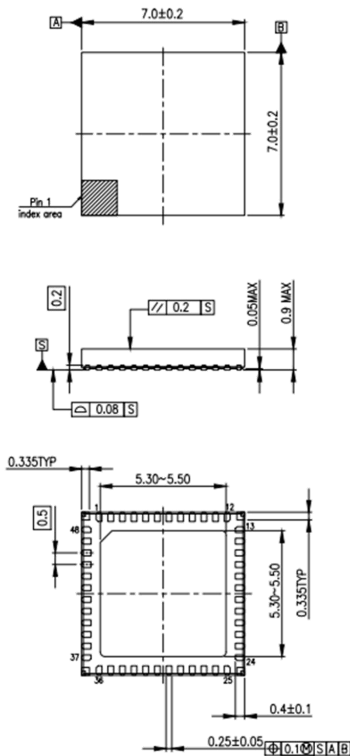
図 12.1 外形寸法図
