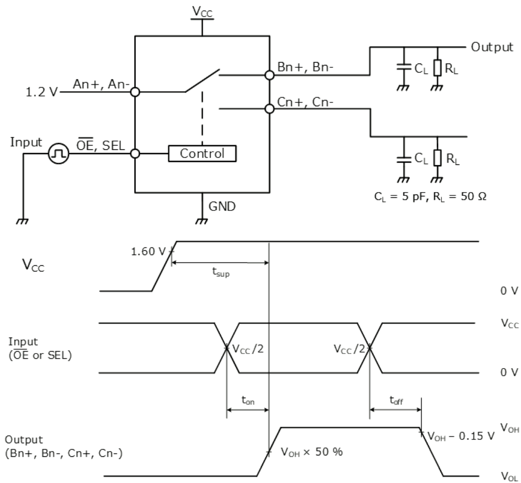
図 13.5 スタートアップ時間, ターンオン時間, ターンオフ時間
