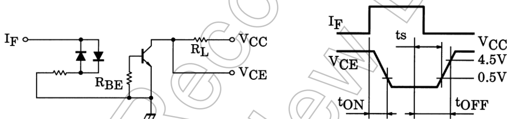
図 1: スwitchング時間測定回路
