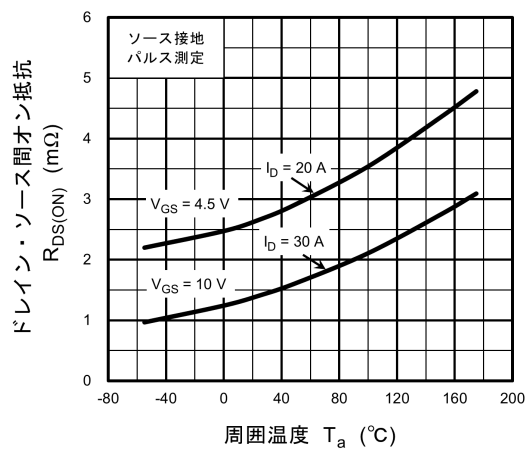
図 8.9 R_{DS(ON)} - T_a
