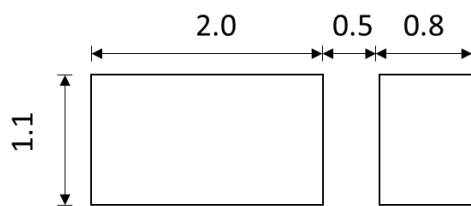
図 9.1 参考パッド寸法(単位: mm)
