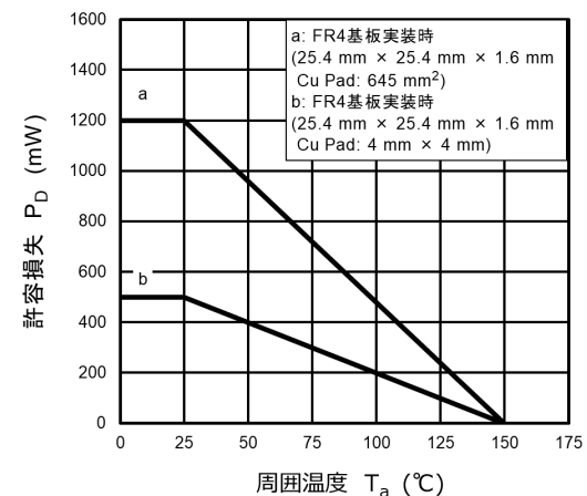
図 10.1.6 P_D - T_a
