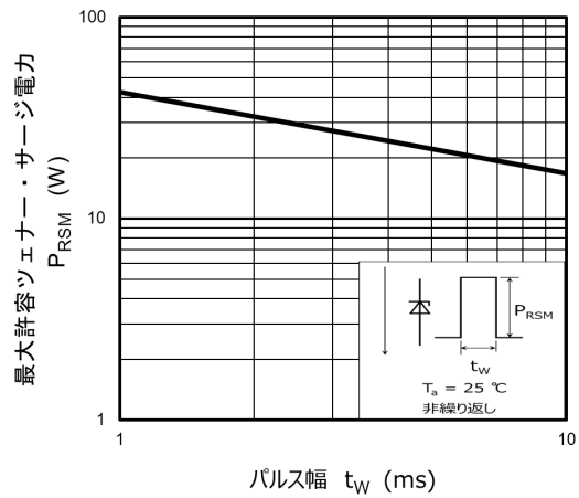
図 10.1.2 P_{RSM} - t_w
