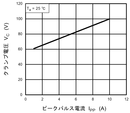
図 10.2.2 V_C - I_{PP}
