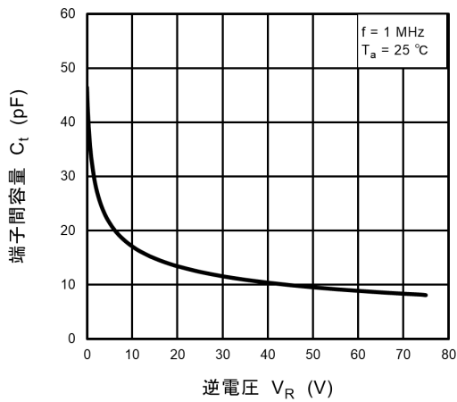
図 10.5.3 C_T - V_R
