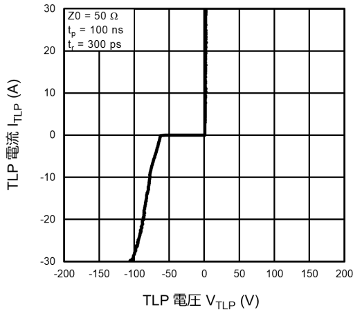
図 10.3.1 I_{TLP} - V_{TLP}
