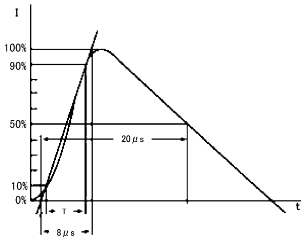
図 10.6.1 V_C - I_{PP} 印加波形 (IEC61000-4-5準拠 8/20 \mu\text{s} pulse)
