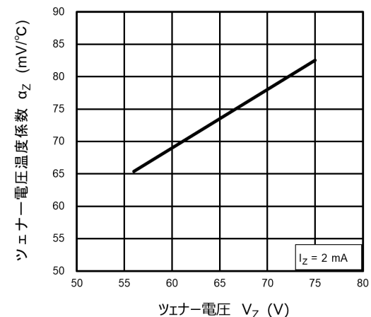
図 10.1.4 \alpha_Z - V_Z
