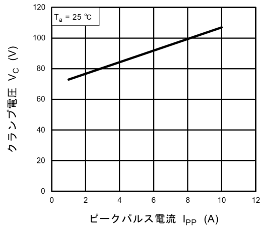
図 10.4.2 V_C - I_{PP}
