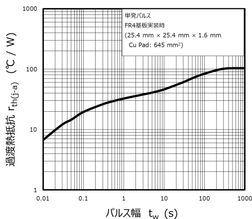
図 10.1.5 r_{th(j-a)} - t_w
