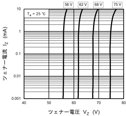
図 10.1.1 I_Z - V_Z
