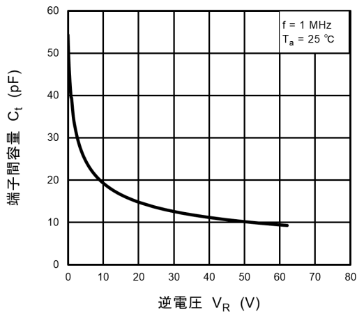
図 10.3.3 C_T - V_R
