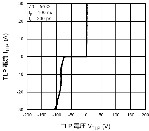
図 10.5.1 I_{TLP} - V_{TLP}
