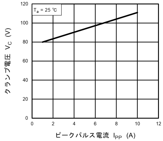
図 10.5.2 V_C - I_{PP}
