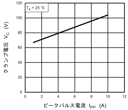
図 10.3.2 V_C - I_{PP}
