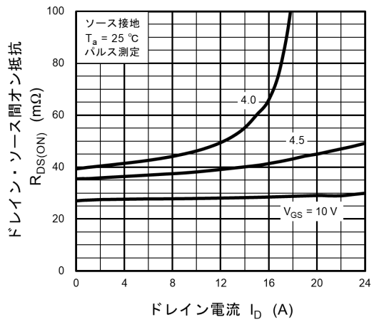
図 8.4 R_{DS(ON)} - I_D
