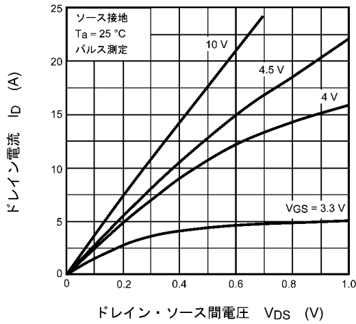
図 8.1 I_D - V_{DS}
