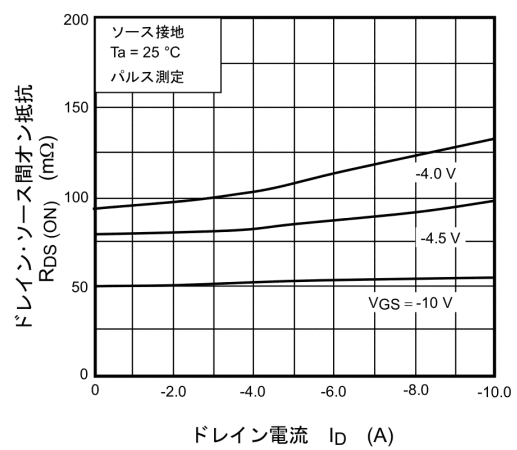
図 8.4 R_{DS(ON)} - I_D
