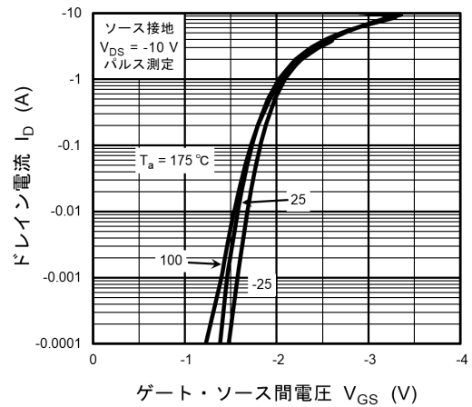
図 8.2 I_D - V_{GS}
