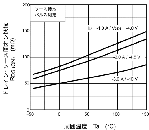
図 8.5 R_{DS(ON)} - T_a
