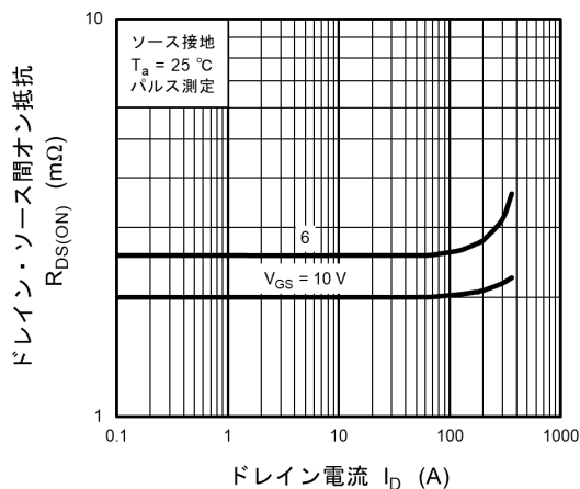
図 8.8 R_{DS(ON)} - I_D
