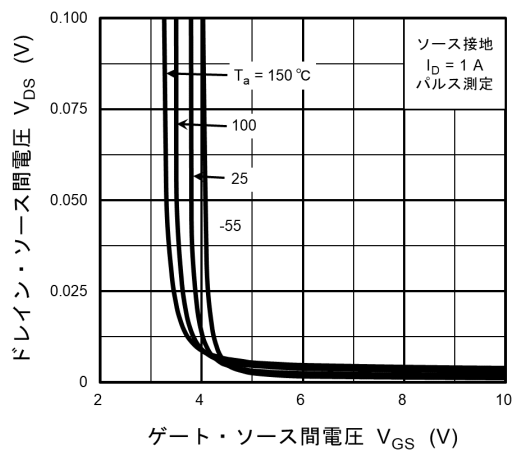
図 8.6 V_{DS} - V_{GS}
