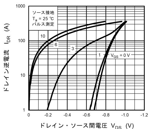
図 8.10 I_{DR} - V_{DS}
