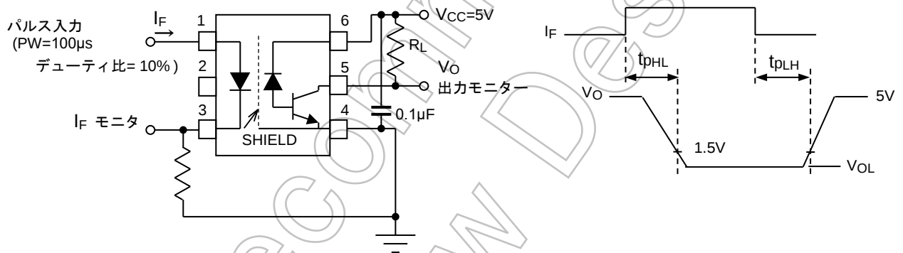
図 1. 伝達遅延時間測定回路、波形
