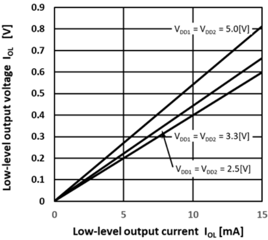
图 13.6. V_{OL} - I_{OL}
