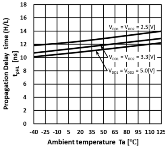
图 13.8. 伝搬遅延 t_{PLH} - T_a
