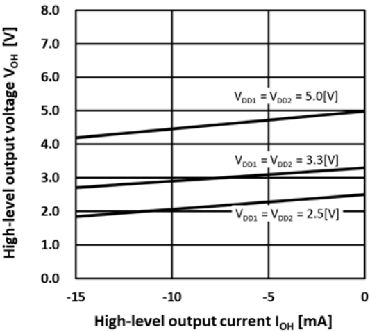
图 13.5. V_{OH} - I_{OH}
