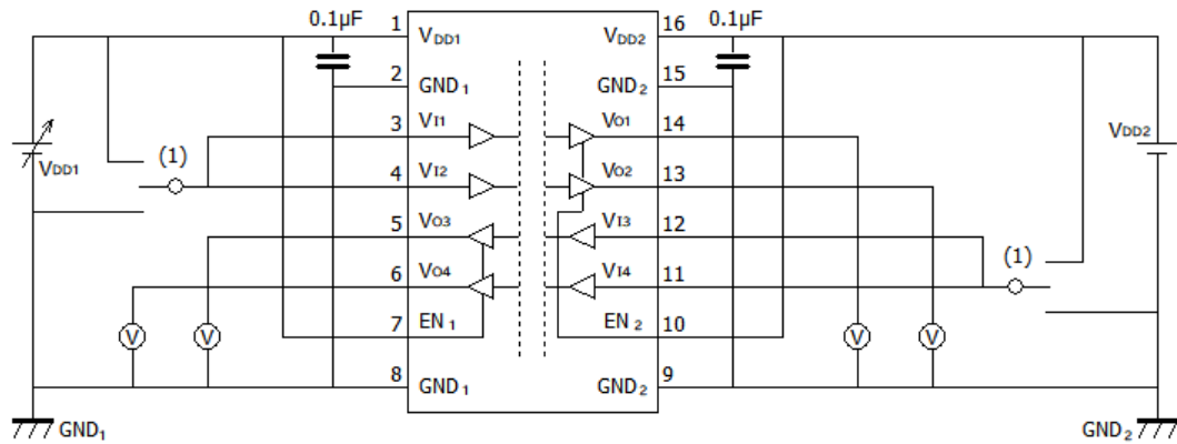
图 12.1.4. DCL542L01A/DCL542H01A V DDIU+/- /V DDIU-/- 特性测定回路图
