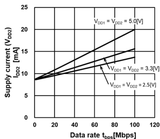
図 13.6. DCL542x01A I_{DD2} 動作電流—データレート
