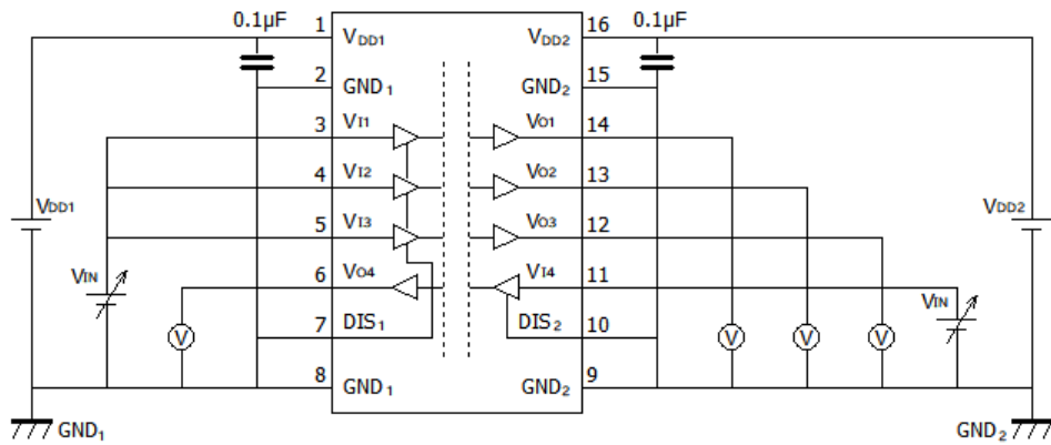
图 12.3.5. DCL541A01A/DCL541B01A V_{IH}/V_{IL} 特性测定回路图
