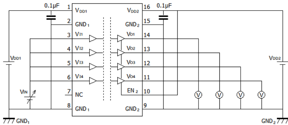
图 12.3.2. DCL540L01A/DCL540H01A V_{IH}/V_{IL} 特性测定回路图
