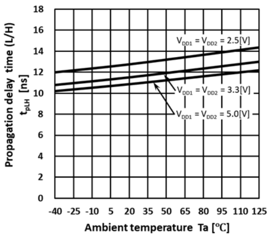
图 13.7. 伝搬遅延 t_{PLH} - T_a
