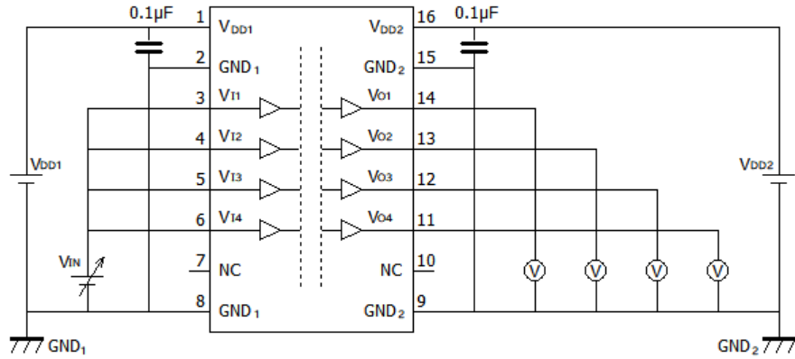
图 12.3.1. DCL540C01A/DCL540D01A V_{IH}/V_{IL} 特性测定回路图
