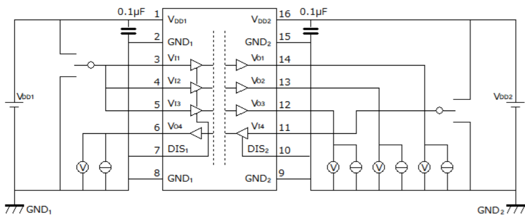
图 12.2.5. DCL541A01A/DCL541B01A V_{OH}/V_{OL} 特性測定回路図
