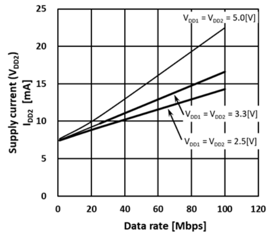
図 13.4. DCL541x01A I_{DD2} 動作電流—データレート
