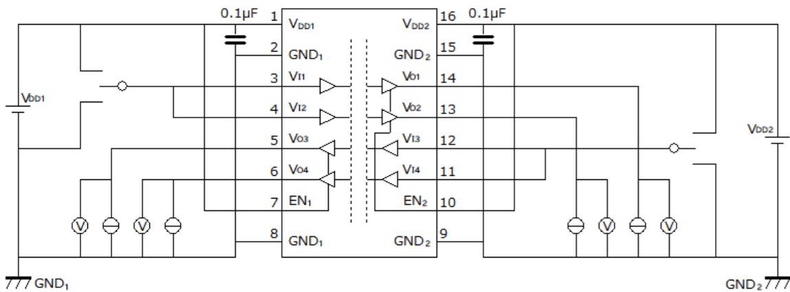
图 12.2.4. DCL542L01A/DCL542H01A V_{OH}/V_{OL} 特性測定回路図
