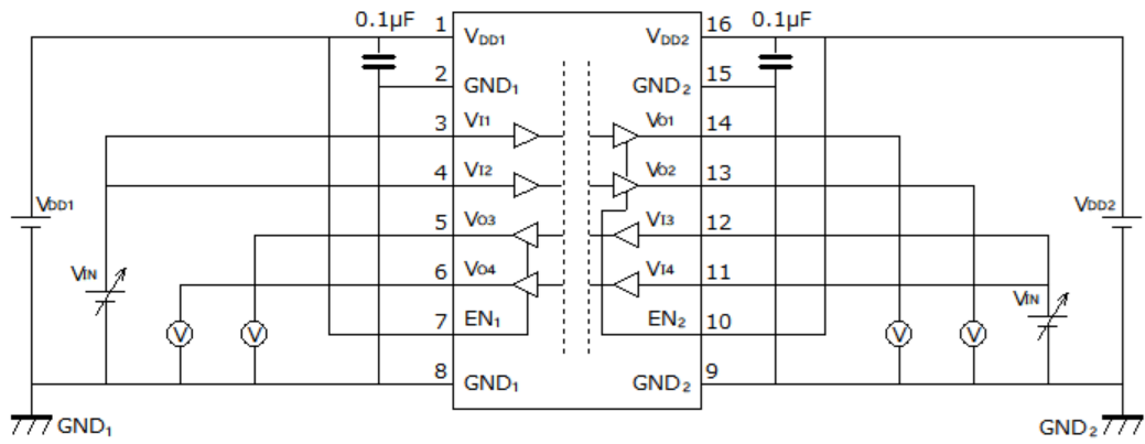
图 12.3.4. DCL542L01A/DCL542H01A V_{IH}/V_{IL} 特性测定回路图
