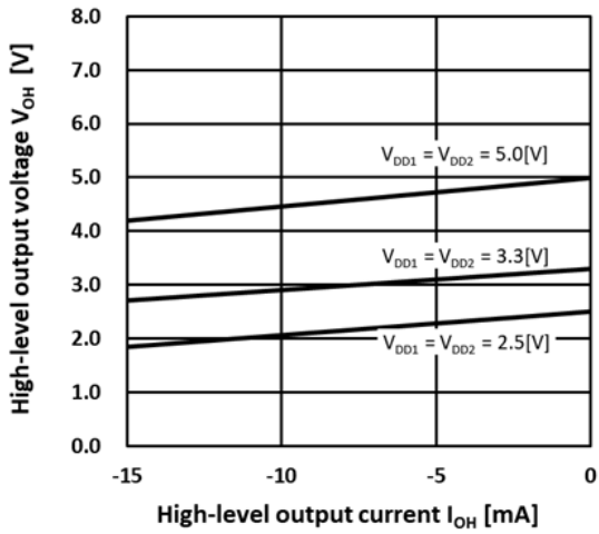
图 13.5. V_{OH} - I_{OH}
