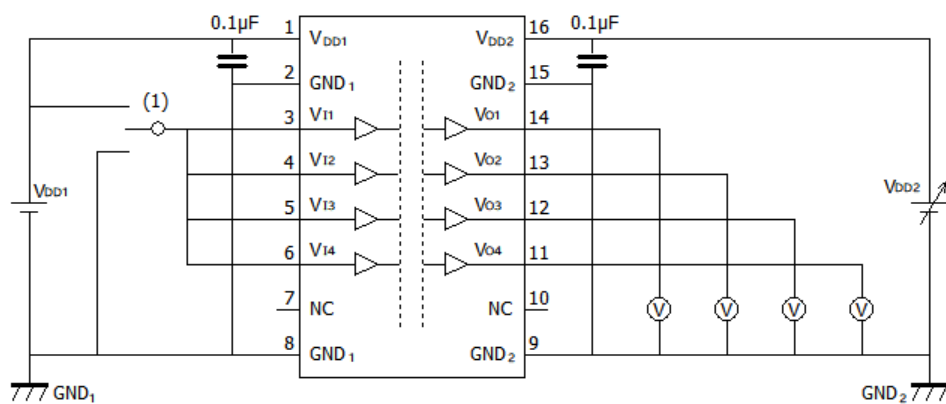
图 12.1.6. DCL540C01A/DCL540D01A V DD2UV+/- /V DD2UV-/- 特性测定回路图
