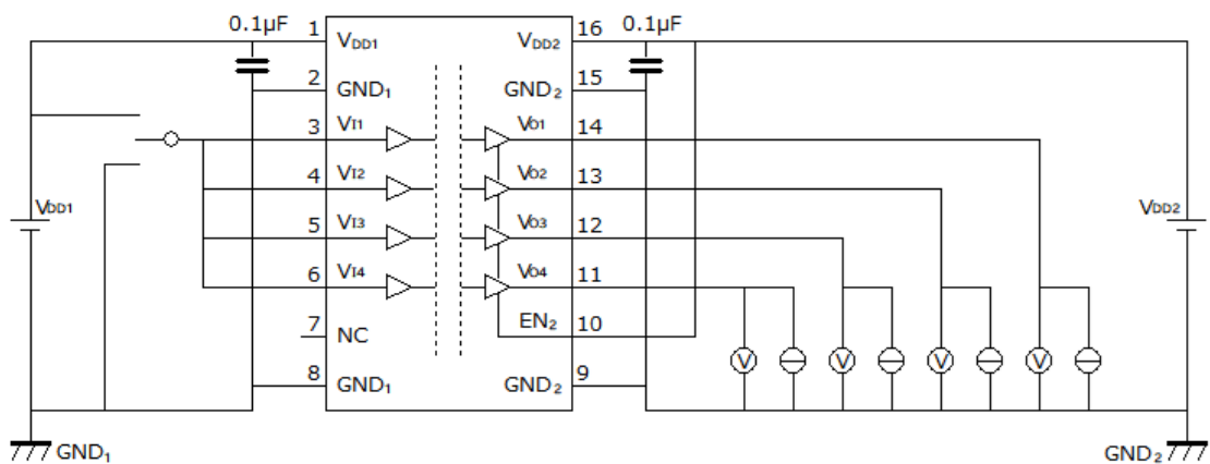
图 12.2.2. DCL540L01A/DCL540H01A V OH /V OL 特性測定回路図
