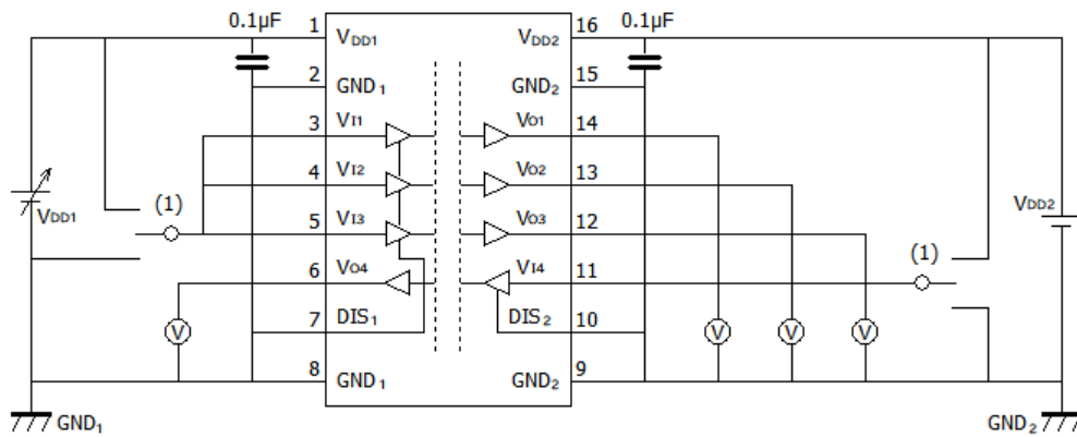
图 12.1.5. DCL541A01A/DCL541B01A V DDIU+/- /V DDIU-/- 特性测定回路图
