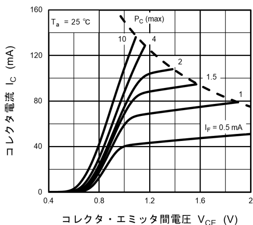
図 12.7 I_C - V_{CE}
