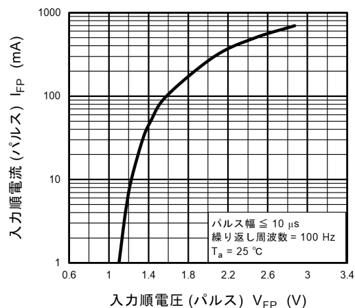
図 12.6 I_{FP} - V_{FP}
