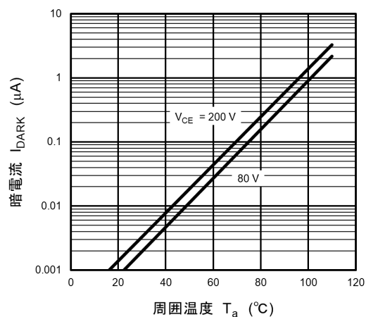
図 12.8 I_{\text{DARK}} - T_a
