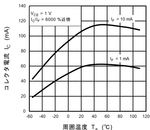
図 12.12 I_C - T_a
