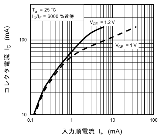
図 12.10 I_C - I_F
