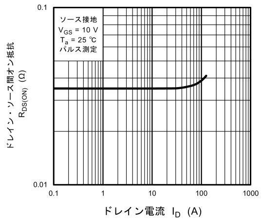
図 8.6 R_{DS(on)} - I_D
