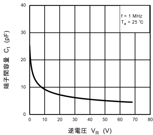
図 10.4.3 C_T - V_R
