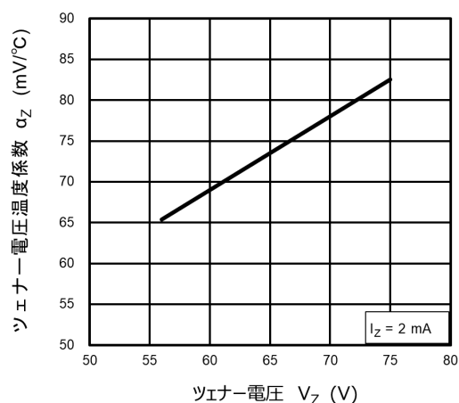
図 10.1.4 \alpha_Z - V_Z
