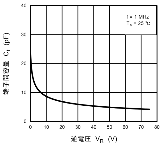
図 10.5.3 C_T - V_R
