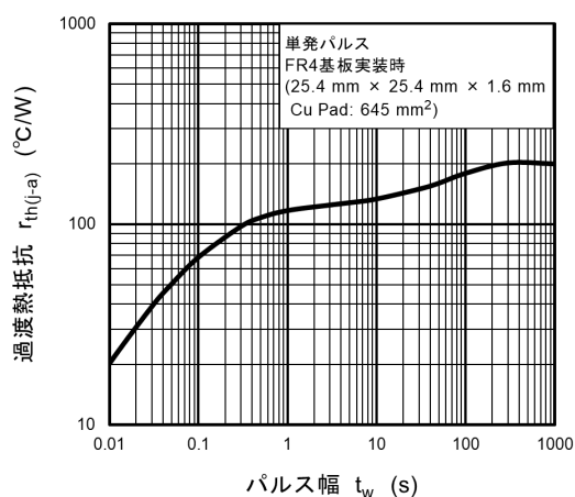
図 10.1.5 r_{th(j-a)} - t_W
