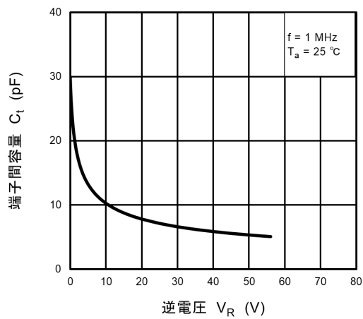
図 10.2.3 C_T - V_R
