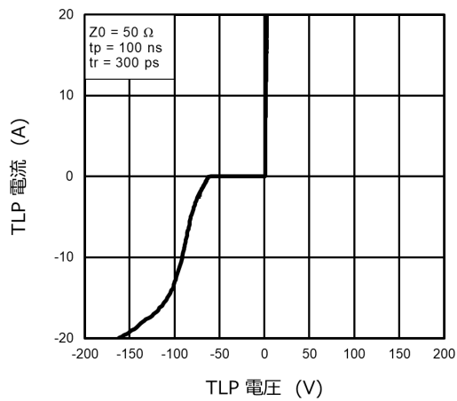
図 10.4.1 I_{TLP} - V_{TLP}
