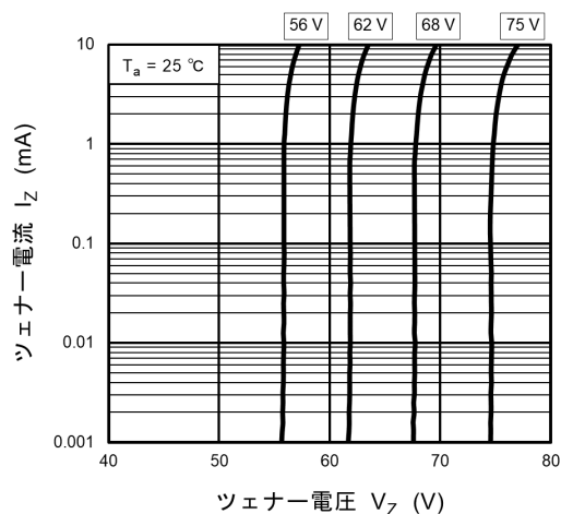
図 10.1.1 I_Z - V_Z(1)
