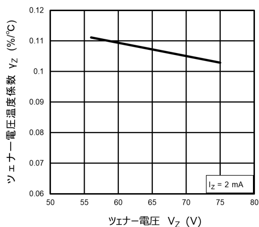
図 10.1.3 Y_Z - V_Z
