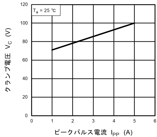
図 10.3.2 V_C - I_{PP}
