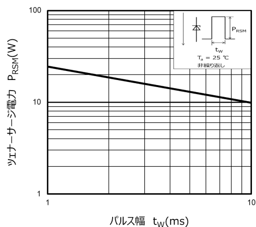
図 10.1.2 P_{RSM} - t_W
