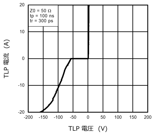
図 10.2.1 I_{TLP} - V_{TLP}
