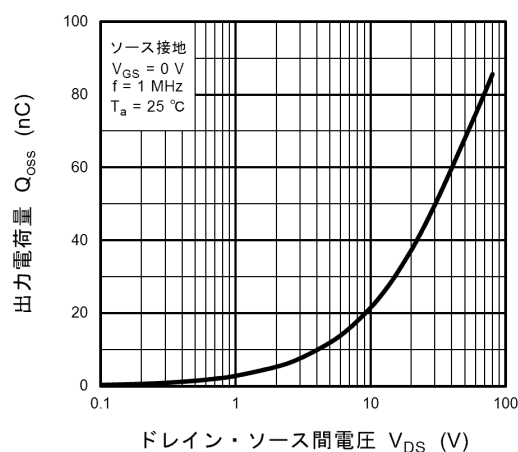
図 8.12 Q_{oss} - V_{DS}
