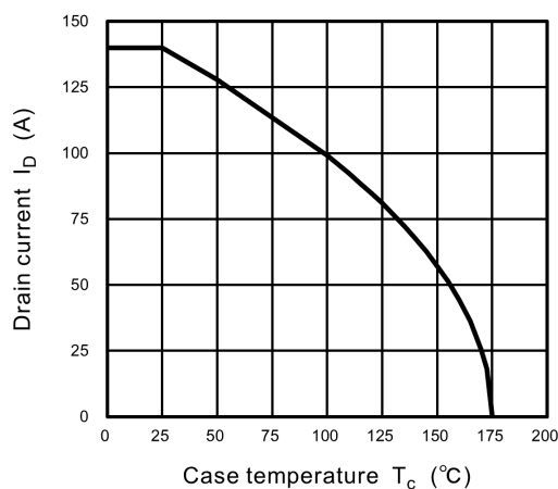
Fig. 8.15 I_D - T_c
