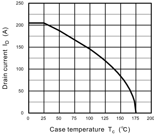
Fig. 8.15 I_D - T_c
