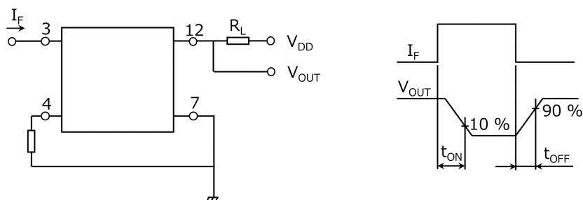
図 11.1 スイッチング時間測定回路, 波形
