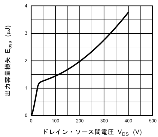
図 8.12 E_{oss} - V_{DS}
