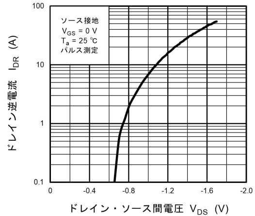
図 8.8 I_{DR} - V_{DS}
