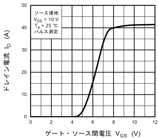
図 8.3 I_D - V_{GS}
