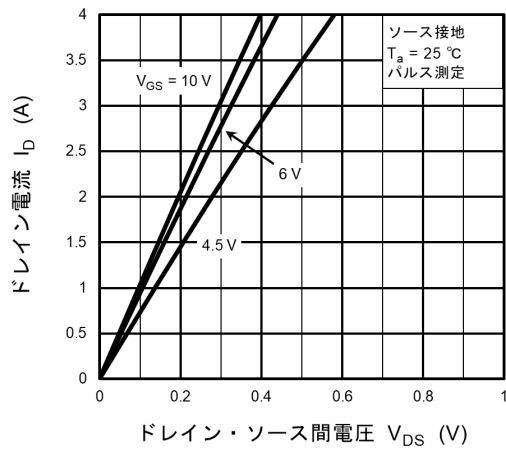
図 9.1 I_D - V_{DS}
