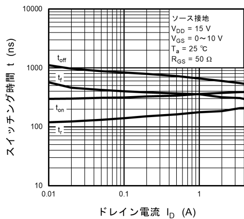
図 9.9 t - I D
