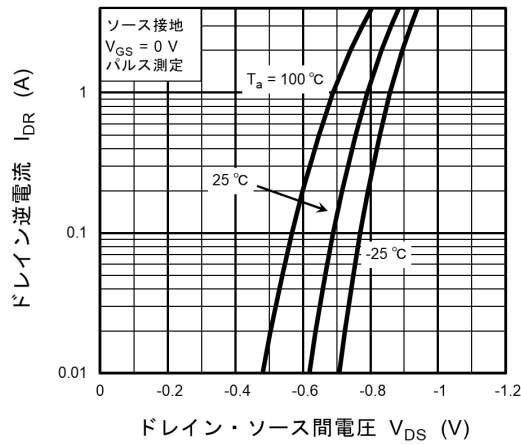
図 9.7 I DR - V DS
