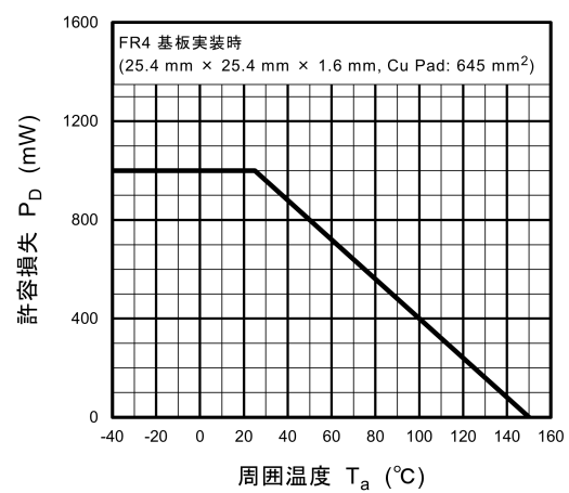
図 9.12 P D - T a
