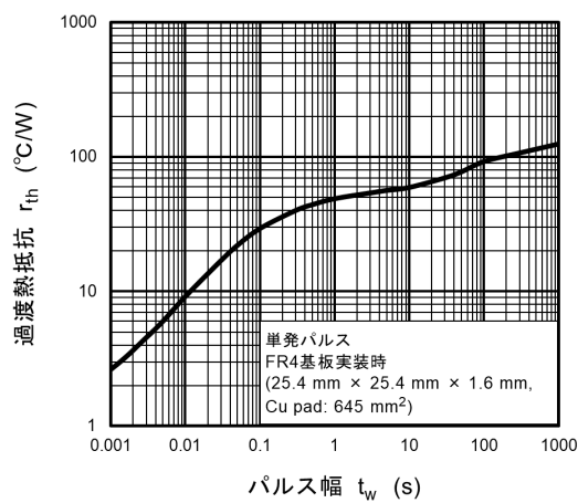
図 9.11 r th - t w
