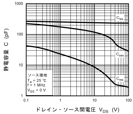
図 9.8 C - V DS
