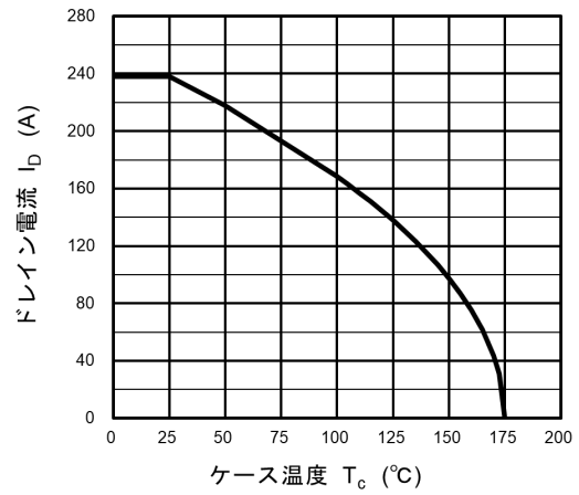
図 8.15 I_D - T_c
