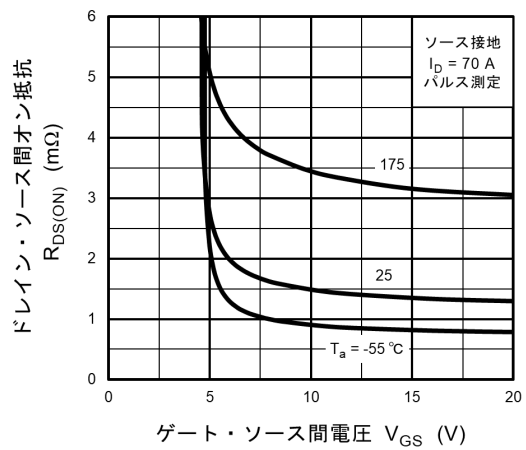
図 8.4 R_{DS(ON)} - V_{GS}
