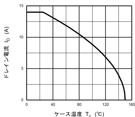
図 8.17 I_D - T_c (最大値 (保証値))
