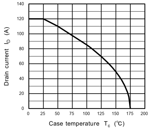
Fig. 8.15 I_D - T_c
