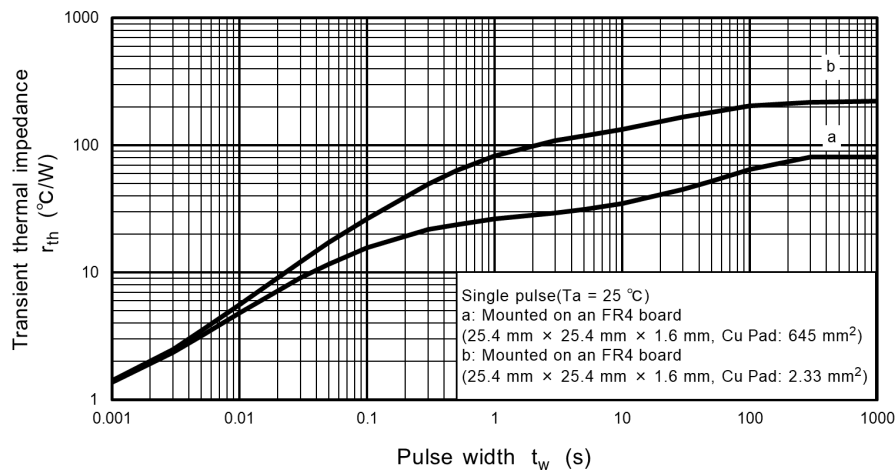
Fig. 7.11 r_{th} - t_w
