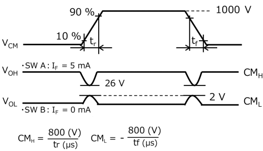
図 13.1.7 コモンモード過渡耐性測定回路, 波形
