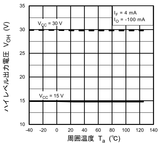
図 13.2.9 V_{OH} - T_a
