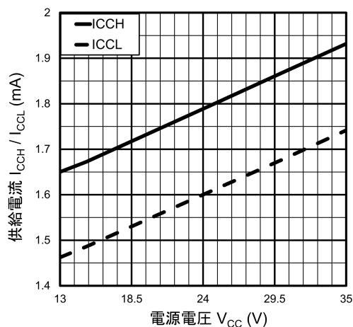
図 13.2.7 I_{CC} - V_{CC}
