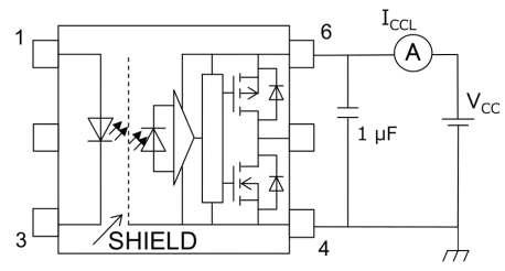
図 13.1.5 I_{CCL} 測定回路
