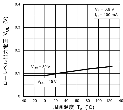
図 13.2.8 V_{OL} - T_a
