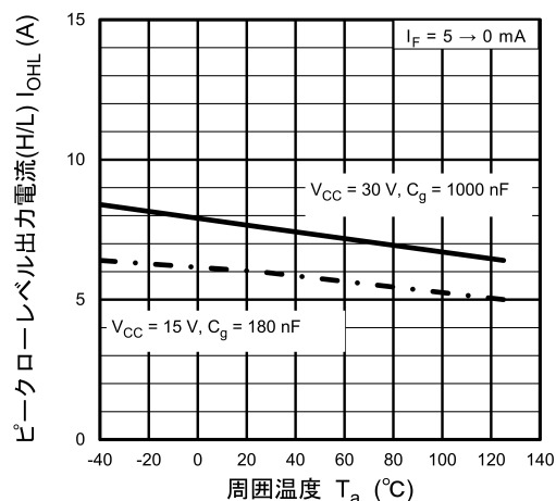
図 13.2.11 I_{OHL} - T_a
