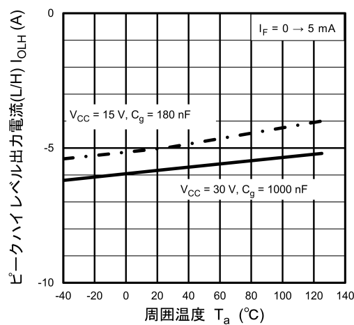
図 13.2.10 I_{OLH} - T_a
