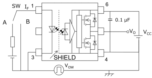
図 13.1.7 コモンモード過渡耐性測定回路, 波形
