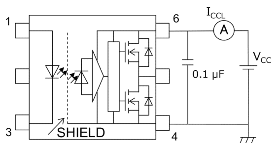
図 13.1.5 ICCCL測定回路
