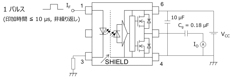
図 13.1.1 IOLH / IOHL測定回路
