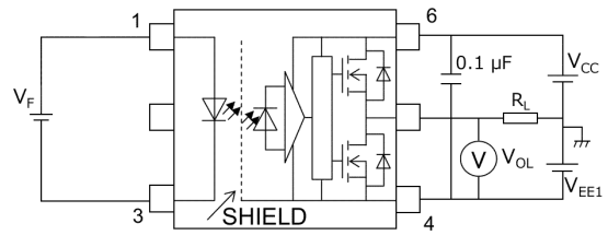
図 13.1.3 VOL測定回路
