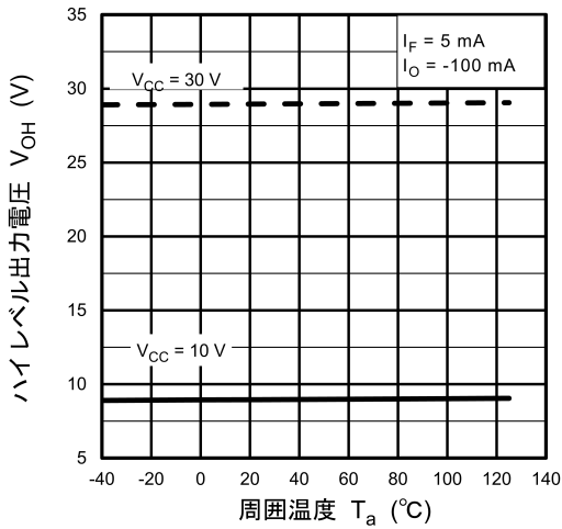
図 13.2.9 V_{OH} - T_a
