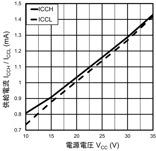
図 13.2.7 I_{CC} - V_{CC}
