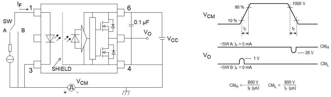
图 13.1.7 コモンモード過渡耐性測定回路, 波形
