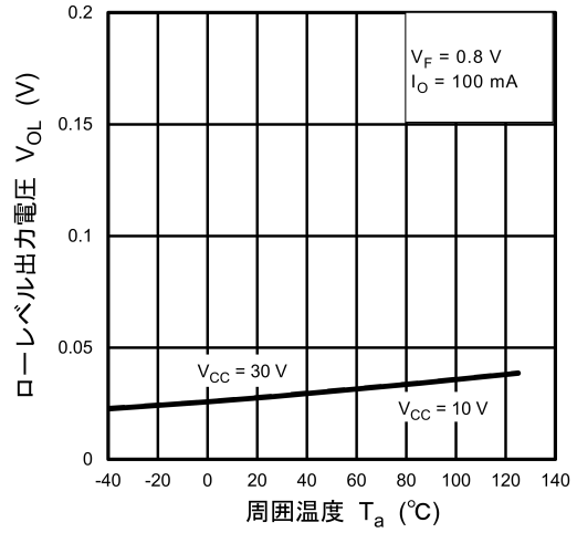
図 13.2.8 V_{OL} - T_a
