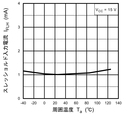
図 13.2.4 I_{FLH} - T_a
