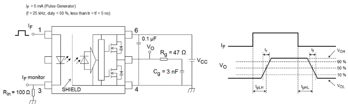
図 13.1.6 伝搬遅延時間測定回路, 波形
