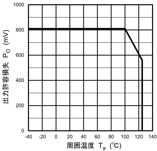
図 13.2.3 P_O - T_a
