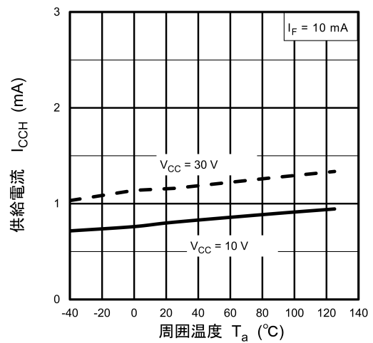
図 13.2.6 I_{CCH} - T_a
