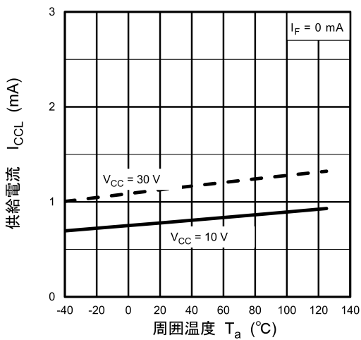
図 13.2.5 I_{CCL} - T_a
