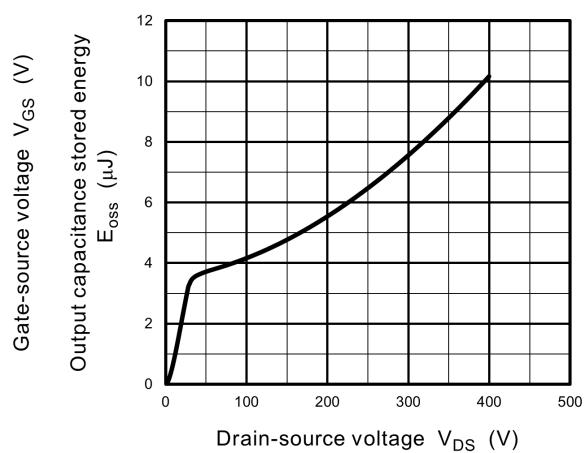
Fig. 8.12 E_{oss} - V_{DS}
