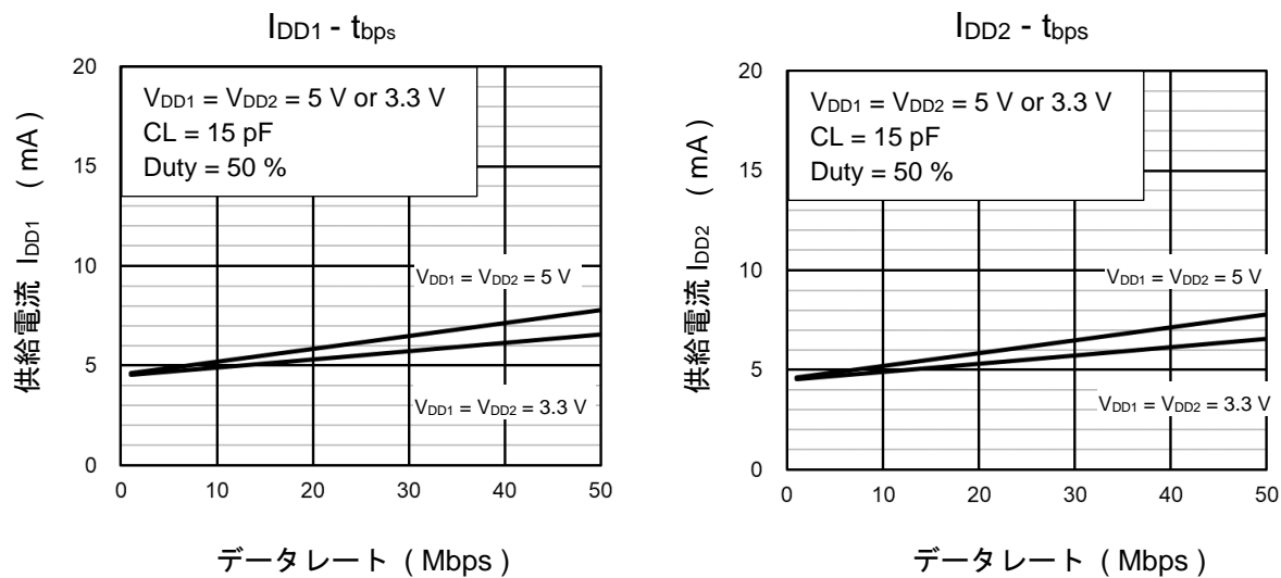
図 12.1 供給電流 - データレート
