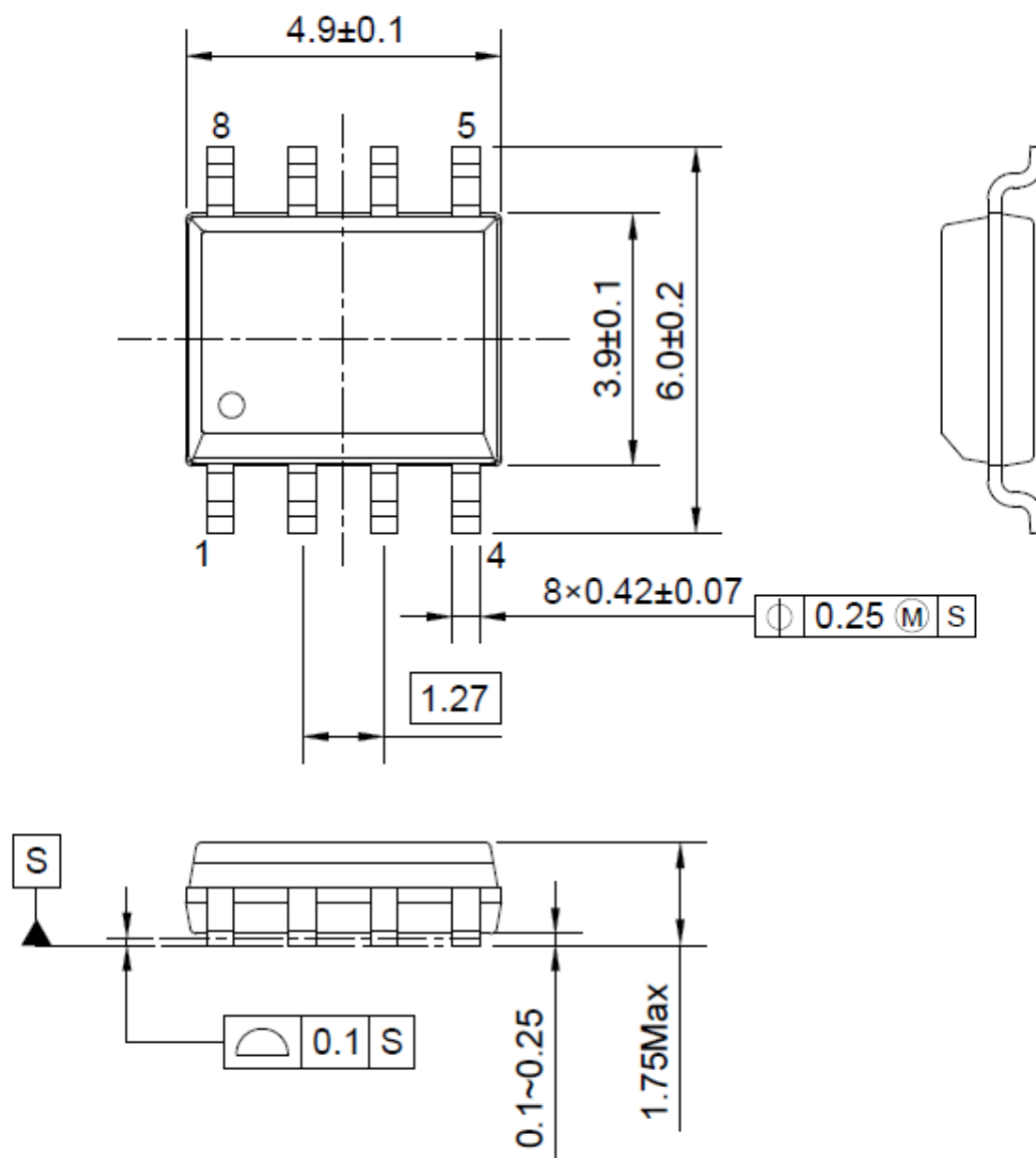
図 14.1 外形寸法図
