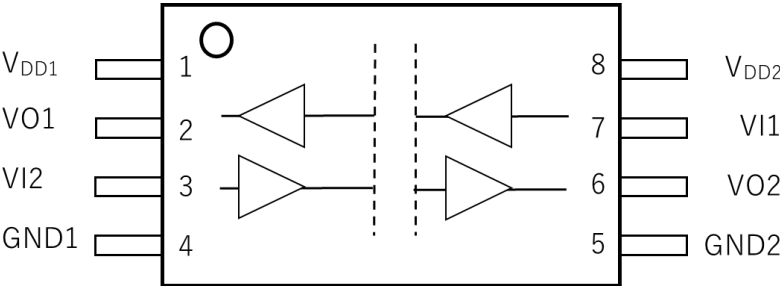
図 6.1 端子配置図 (top view)
