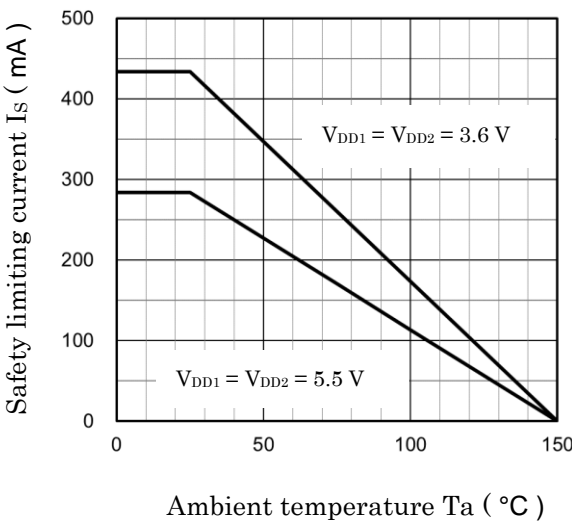
図 9.1 許容電流特性
