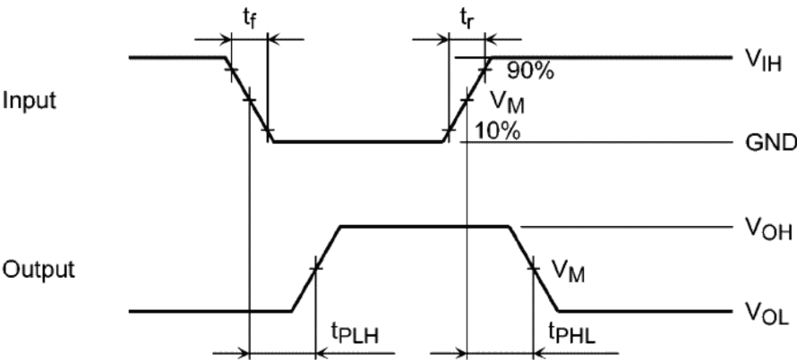
図 9.7.1 t_{PLH}, t_{PHL}
