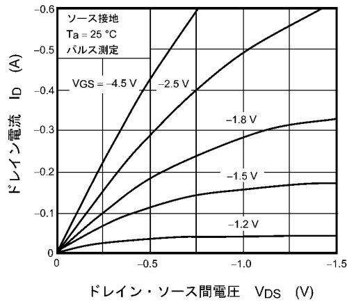
図 8.1 I_D - V_{DS}
