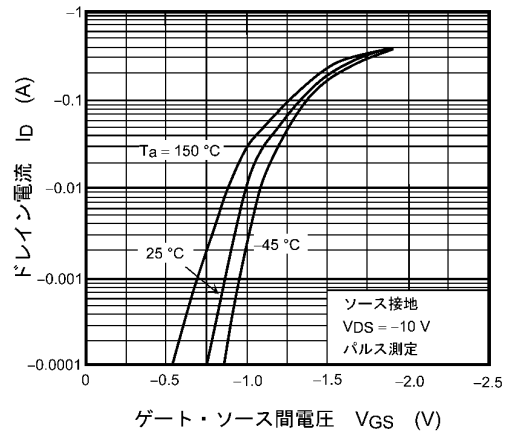
図 8.2 I_D - V_{GS}
