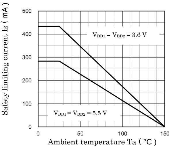
図 9.1 許容電流特性
