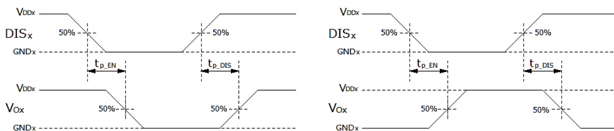
図 8.2 ディセーブル伝搬遅延時間 波形図
