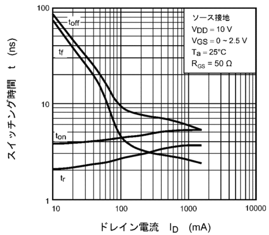
図 7.10 t - I_D
