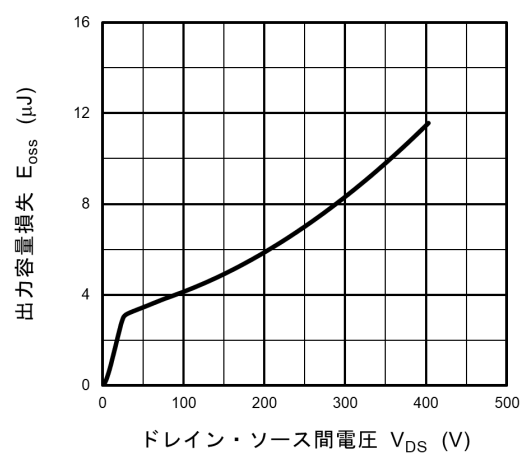
図 8.12 E_{oss} - V_{DS}
