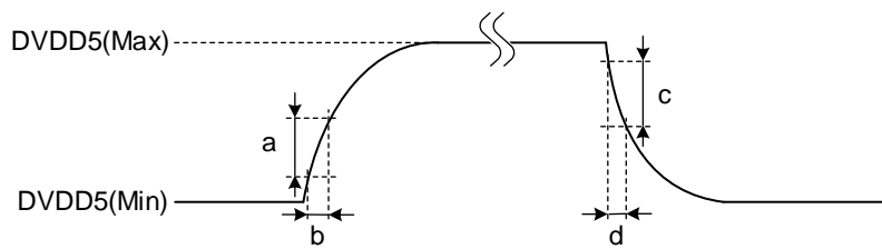
図 7.1 電源変動レート
