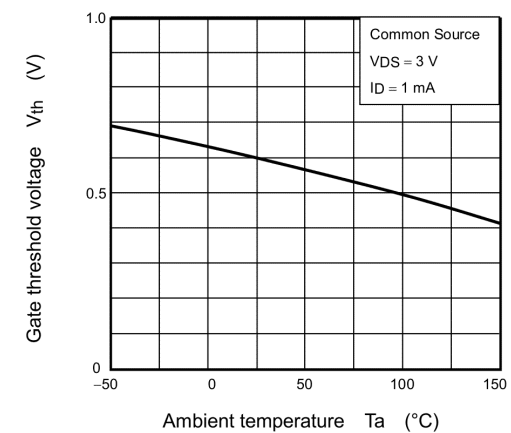
Fig. 7.6 Vth - Ta
