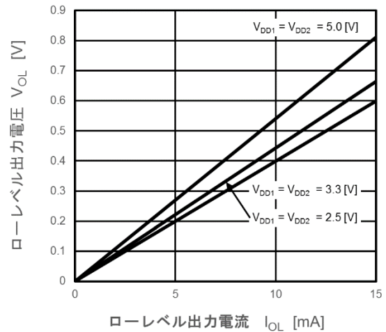
図 13.6 V OL -I OL
