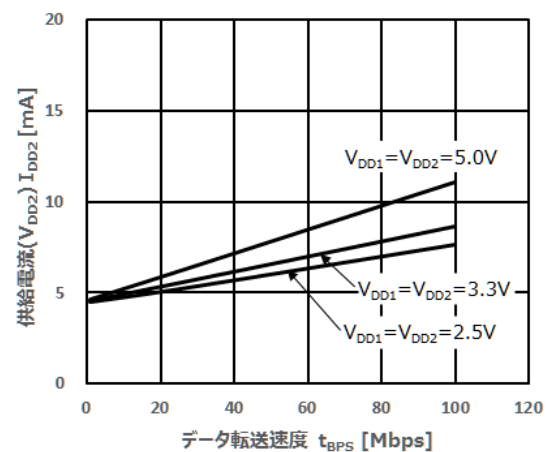
図 13.4 DCL521x00 I DD2 動作電流—データレート
