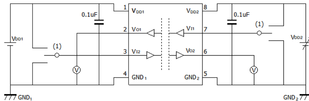
図 12.1.3 DCL520C00/DCL520D00 V DD2UV+ / V DD2UV- 特性測定回路図
