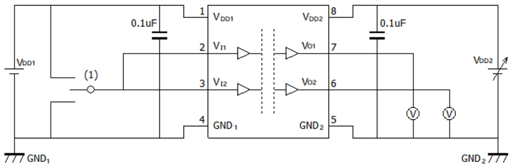
図 12.1.2 DCL521C00/DCL521D00 V DD1UV+ / V DD1UV- 特性測定回路図
