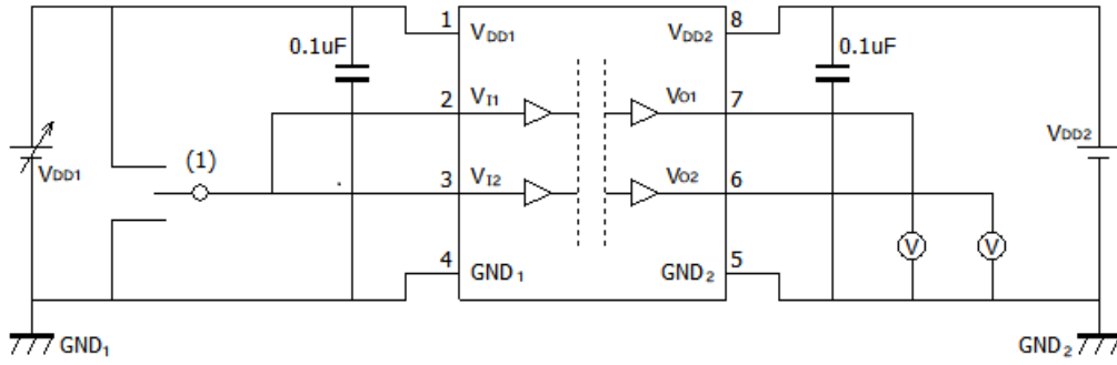
図 12.1.1 DCL520C00/DCL520D00 V DD1UV+ / V DD1UV- 特性測定回路図
