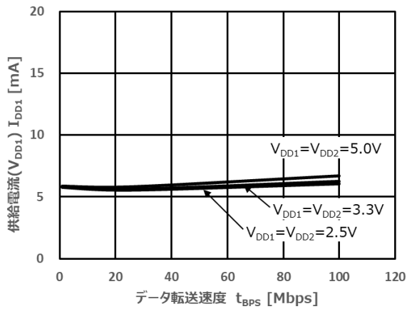
図 13.1 DCL520x00 I DD1 動作電流—データレート
