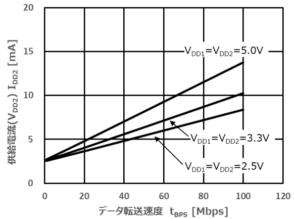
図 13.2 DCL520x00 I DD2 動作電流—データレート
