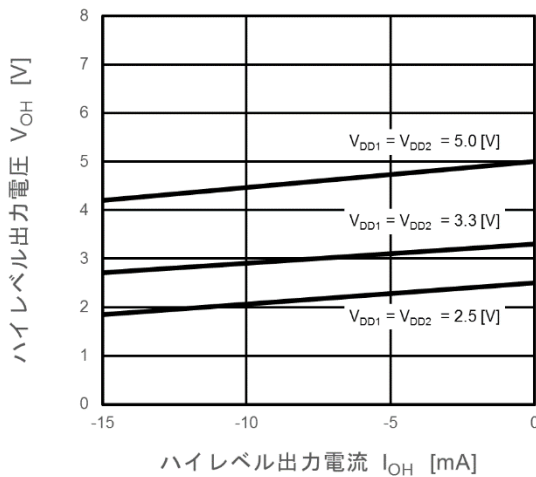
図 13.5 V OH -I OH
