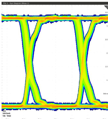
図 14.1 DCL521x00のアイ・ダイアグラム例
