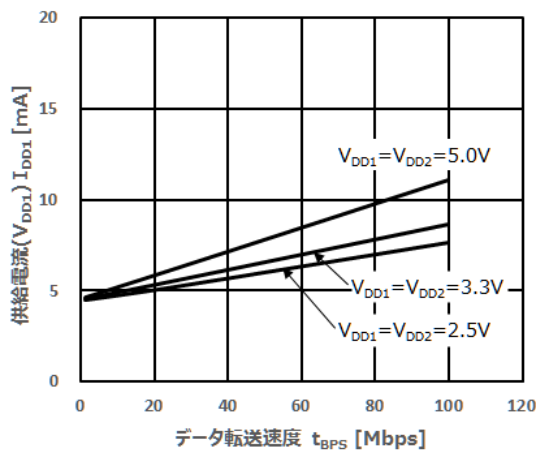
図 13.3 DCL521x00 I DD1 動作電流—データレート
