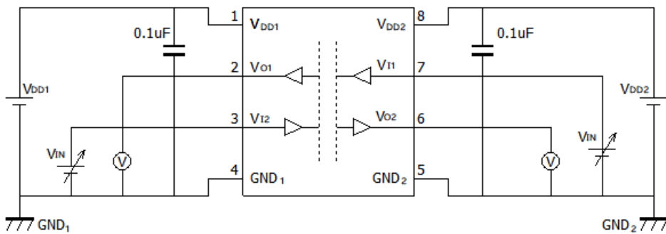
图 12.3.2 DCL521C00/DCL521D00 V_{IH}/V_{IL} 特性测定回路图
