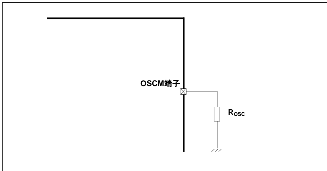
図 10 チョッピング周波数( f_{CHOP} )
