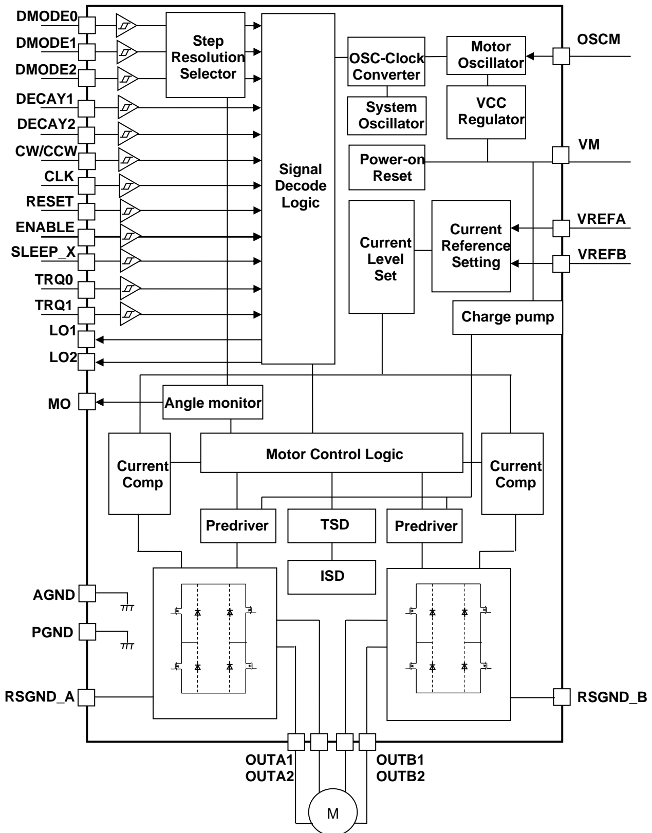
図4 ブロック図
