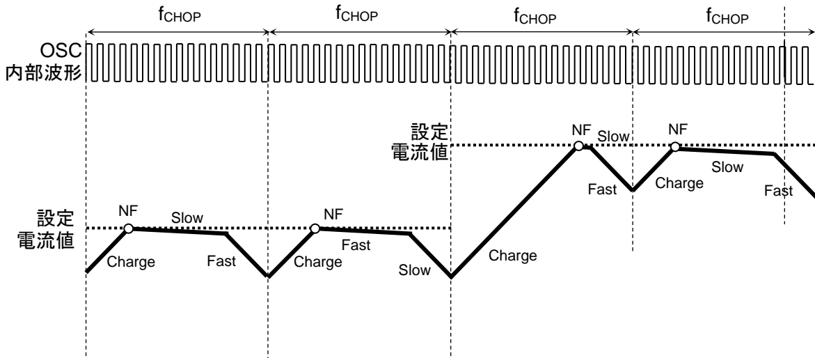
図 7.11.1 設定電流値が増加方向の場合
