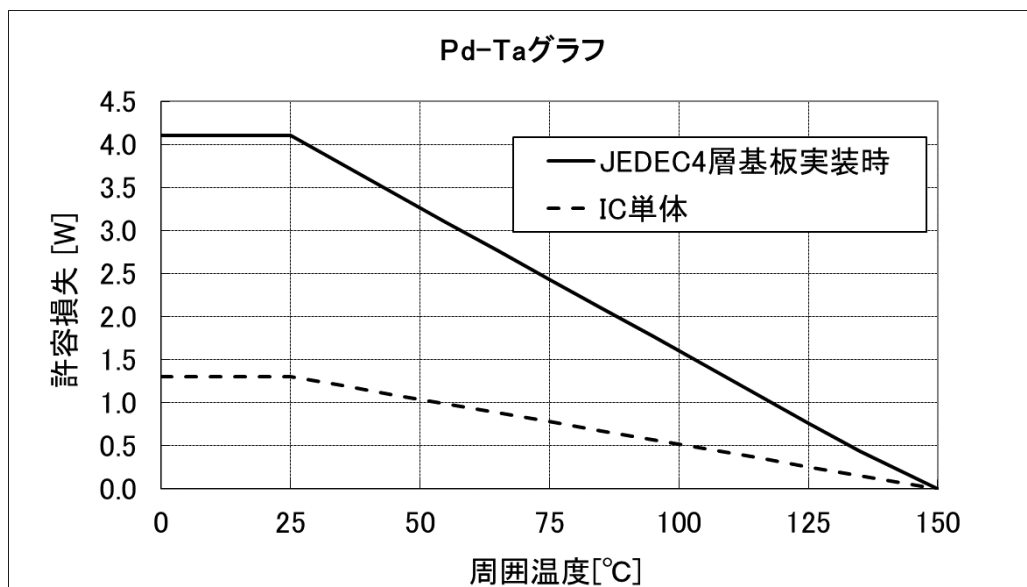
図 16 PD-Ta グラフ
