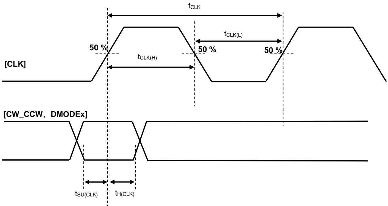
図 20.2 TB67S559FTG(CLK とその他制御信号の関係)
