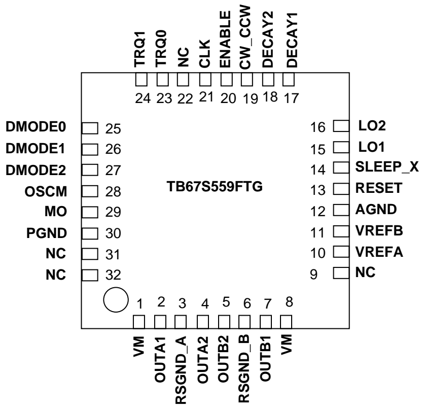
図3 ピン配置図
