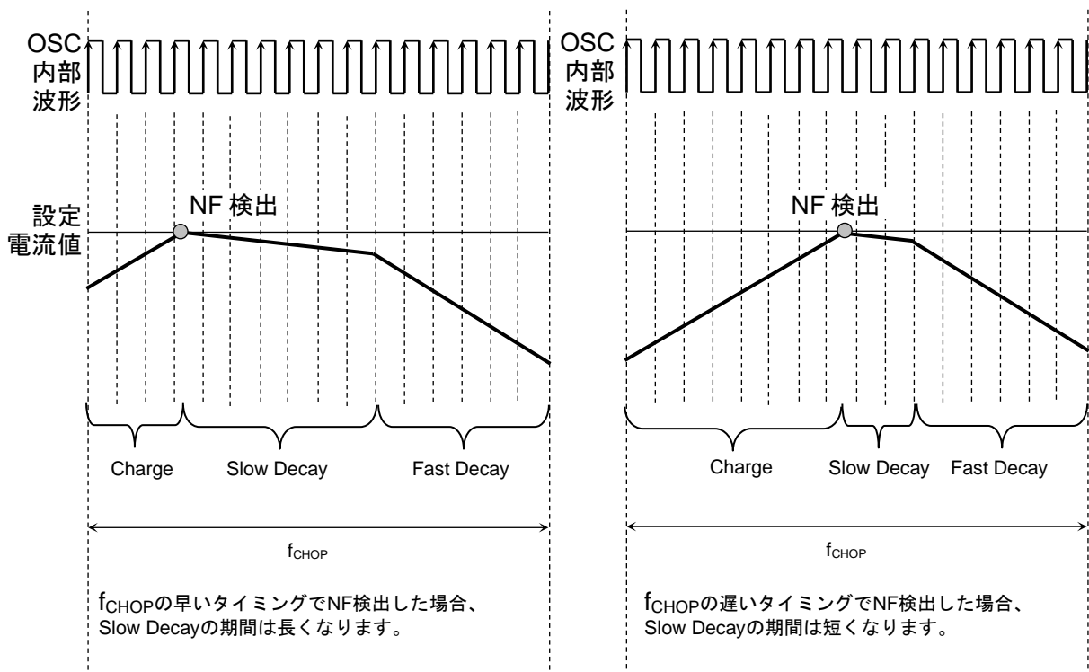
図 7.10 定電流 PWM 動作の各時間
