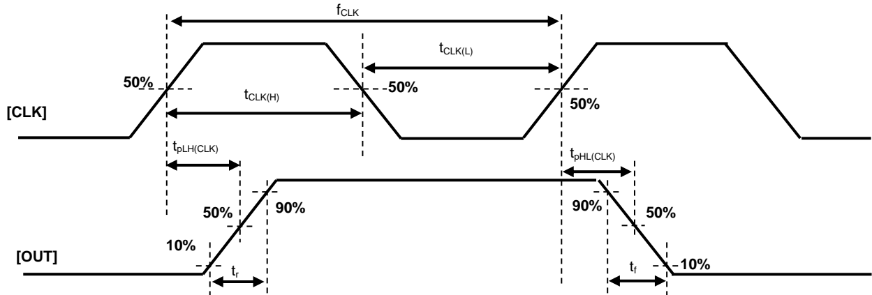
図 20.1 TB67S559FTG(CLK と出力の関係)
