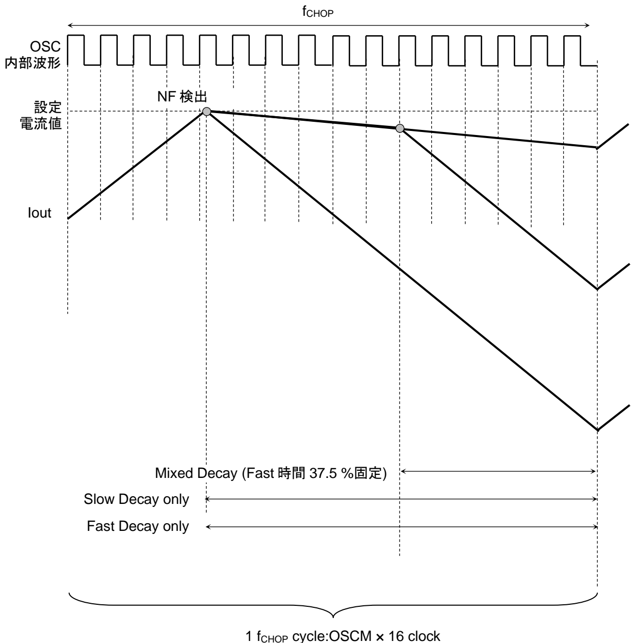
図 7.8 Selectable Mixed Decay ファンクション
