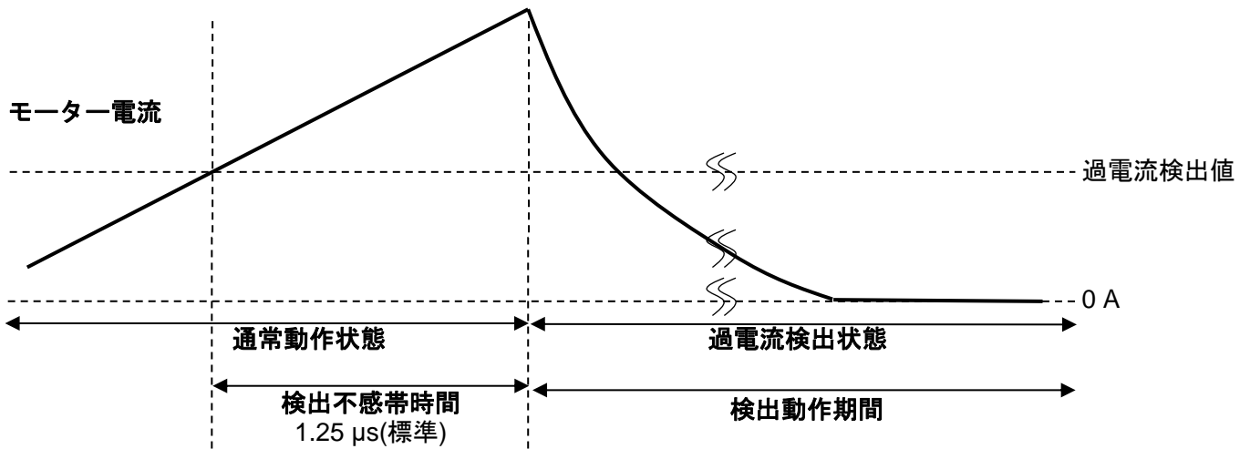
図 14 過電流検出について
