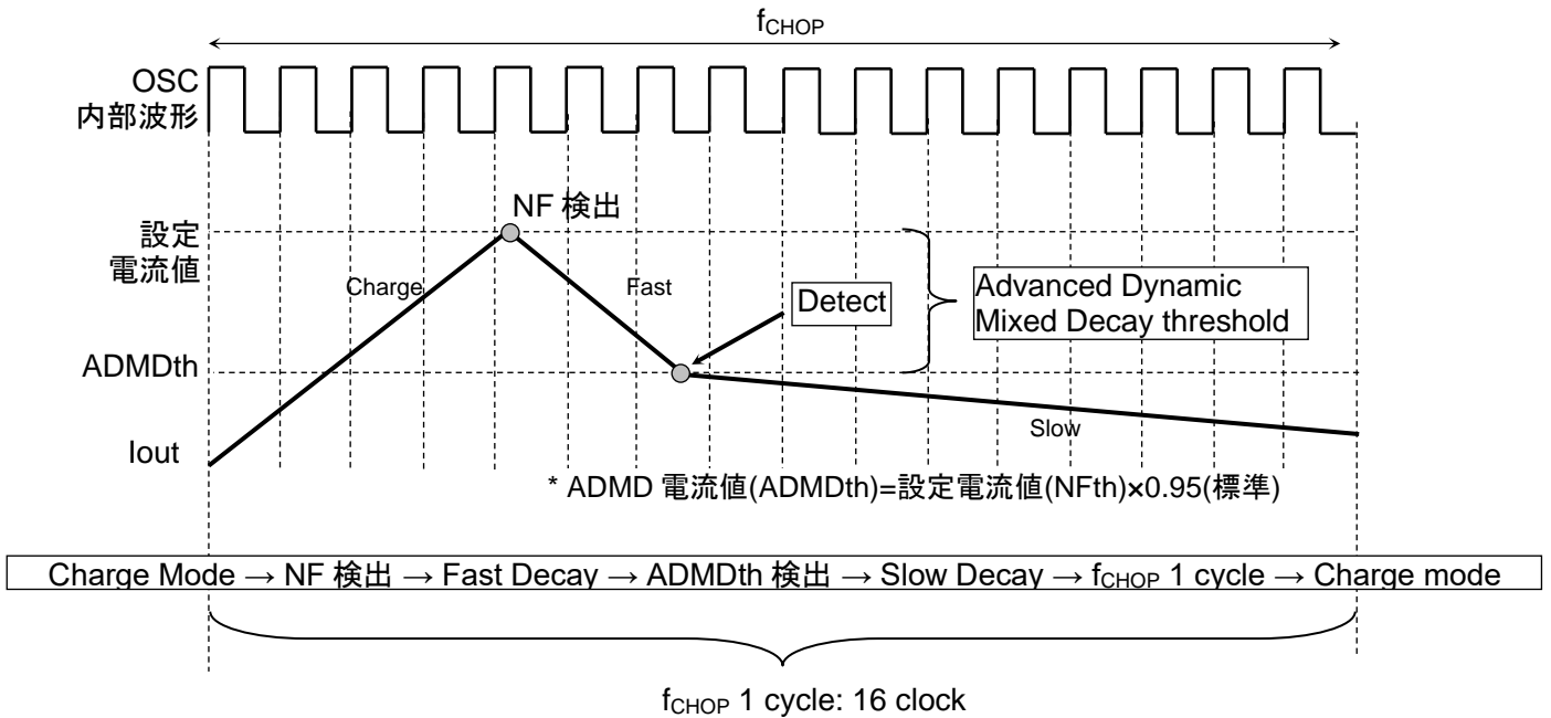
図 7.12.1 ADMD (Advanced Dynamic Mixed Decay) 定電流制御 1
