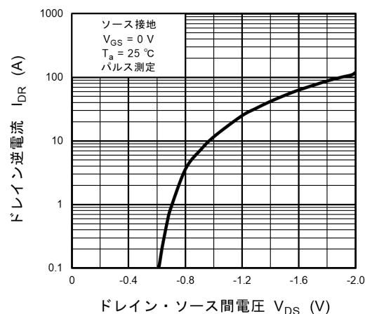
図 8.8 I_{DR} - V_{DS}
