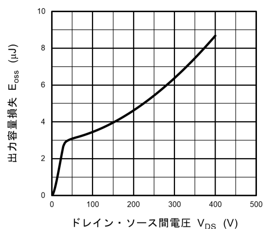
図 8.12 E_{oss} - V_{DS}
