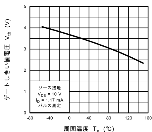
図 8.10 V_{th} - T_a
