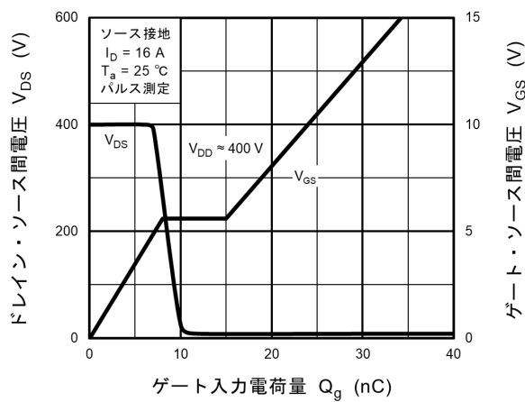
図 8.11 ダイナミック入出力特性
