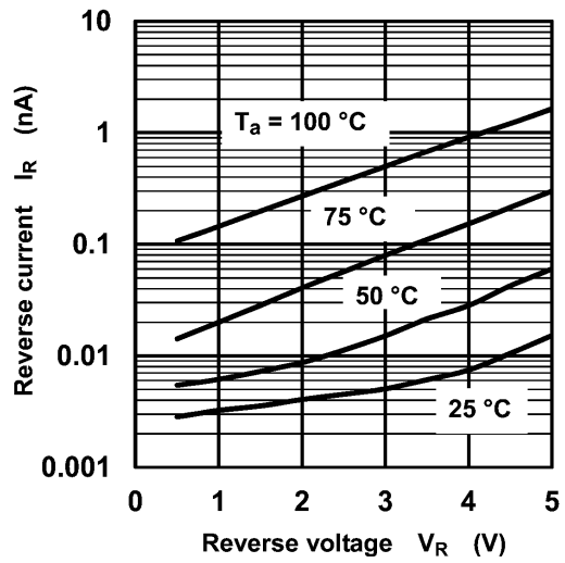
図 7.2 I_R - V_R
