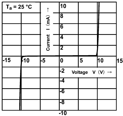
図 7.1 I - V
