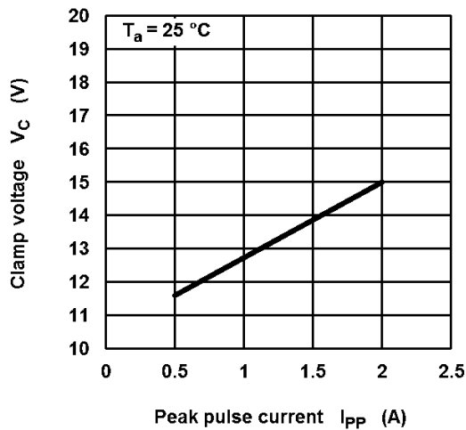
図 8.1 V_C - I_{PP}
