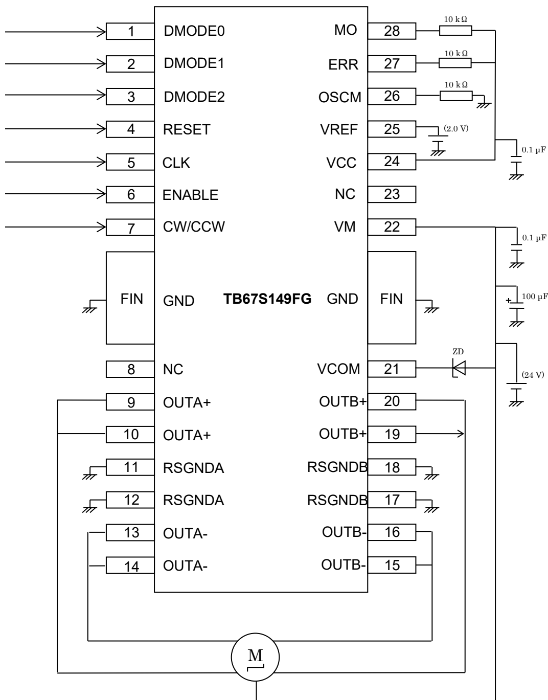
図 10.1 応用回路例
