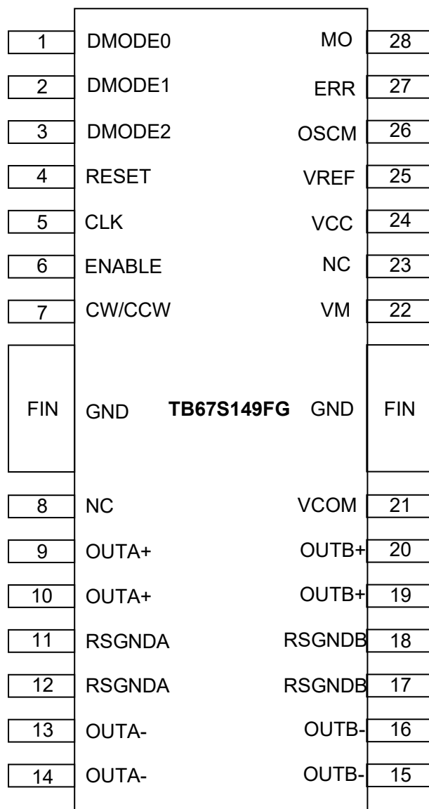
図 4.1 端子配置図
