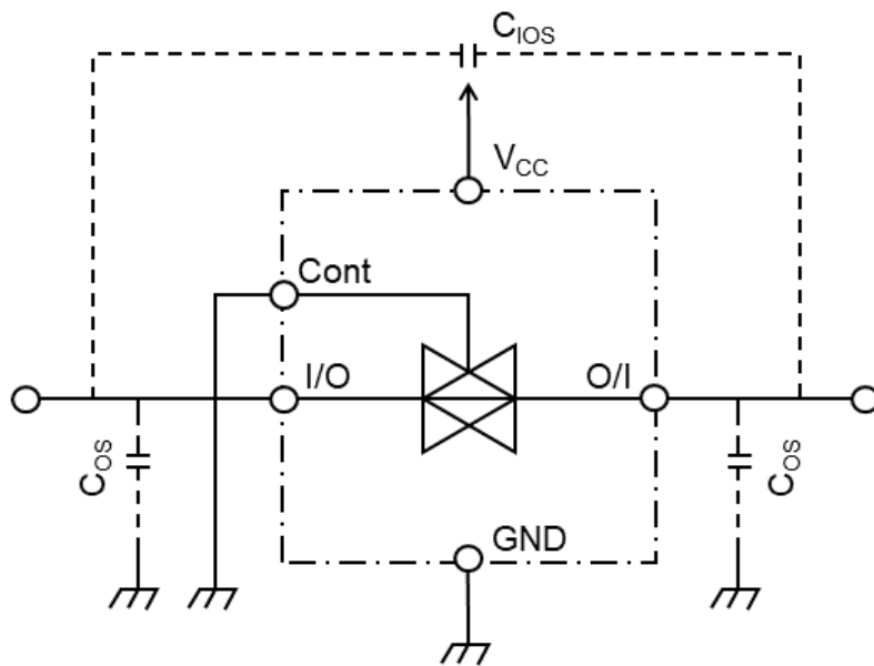
図 2 C_{ios} , C_{os}
